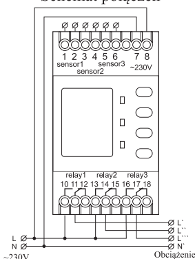
Schemat połączeń
