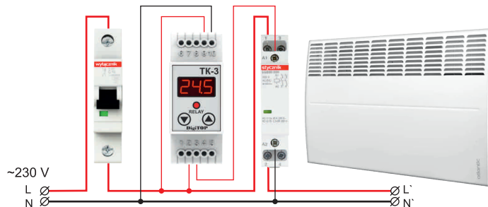
Przykład sterowania ogrzewaniem z wykorzystaniem termoregulatora TK-3
