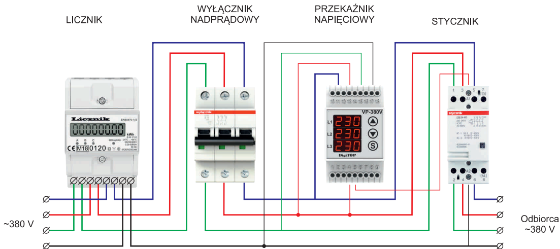
Zabezpieczenie odbiorców 3-fazowych
