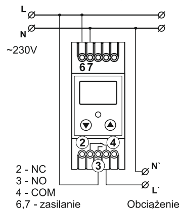
Schemat połączeń
