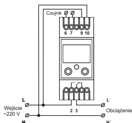
Schemat połączeń
