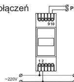
Schemat połączeń
